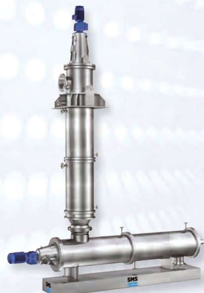
Комбинированные сушильные аппараты
