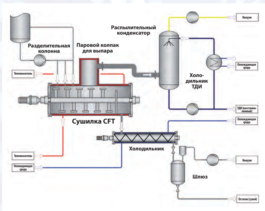
Технология регенерации ТДИ
