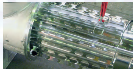
Деталь ротора
